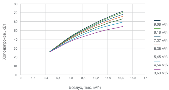
60 кВт: холодопроизводительность при разных расходах воды
