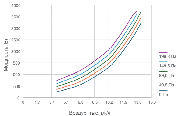
60 кВт: мощность вентиляторов при разных Др
