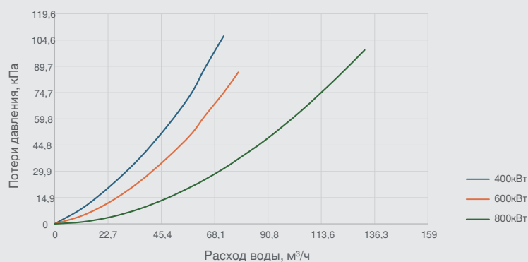
Расход воды и потери давления
