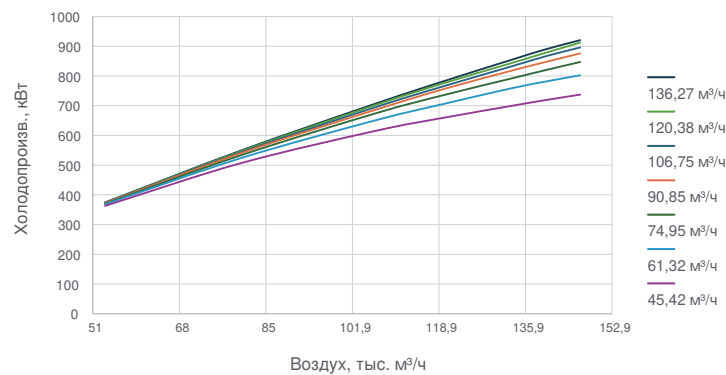
800 кВт: холодопроизводительность при разных расходах воды
