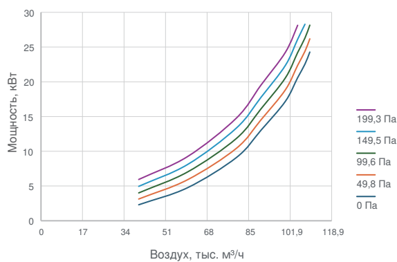
800 кВт: мощность вентиляторов при разных Др
