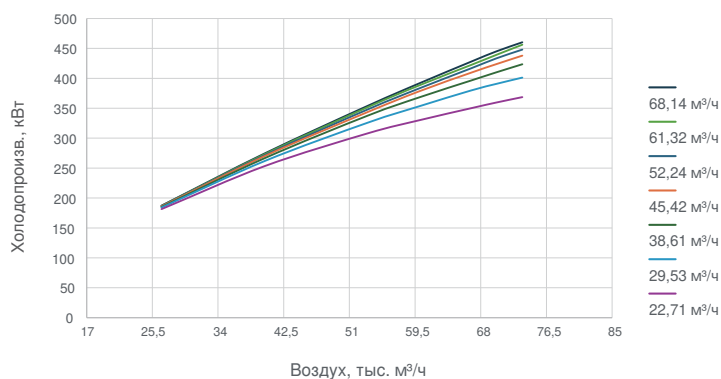
400 кВт: холодопроизводительность при разных расходах воды
