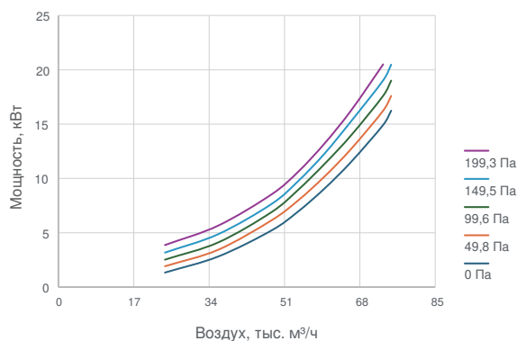
400 кВт: мощность вентиляторов при разных Др
