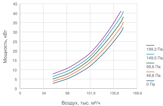
800 кВт: мощность вентиляторов при разных Др
