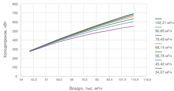
800 кВт: холодопроизводительность при разных расходах воды
