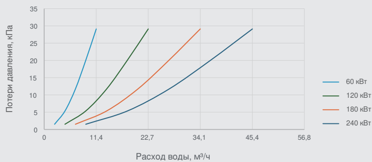
Расход воды и потери давления
