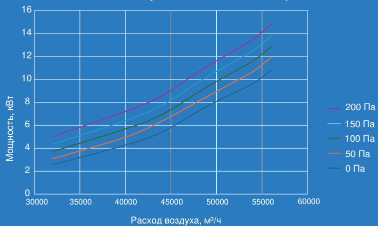
Расход воздуха и мощность вентиляторов
