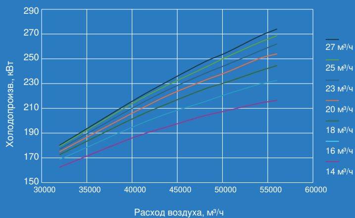
Расход воздуха и холодопроизводительность
