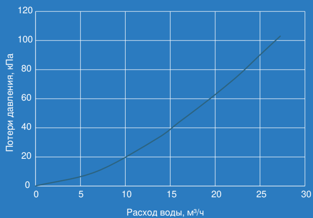
Расход воды и потери давления
