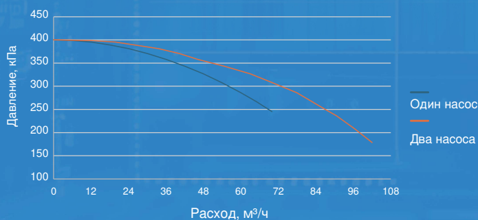
Вторичный контур: расход и давление
